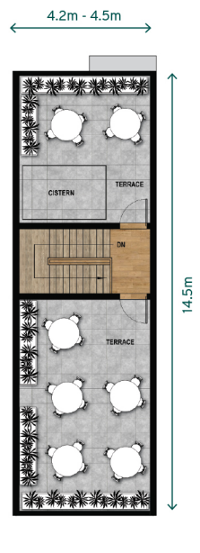
ជាន់ដំបូល - Roof Floor
